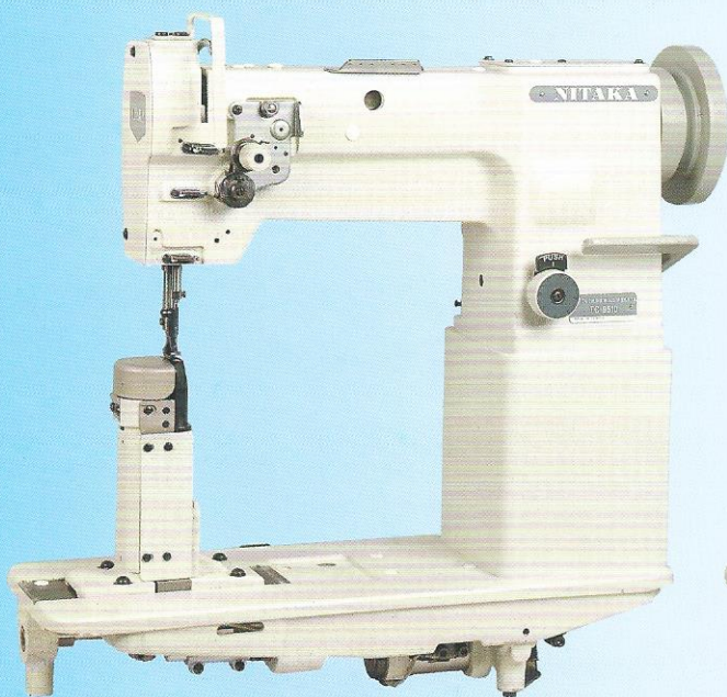
TC-9510 左梭座 LEFT-SIDE POSTBED POSTE LADO IZQUIERDO TC-9510L 可適用於#0線 ACCEPTABLE #0 THREAD ACEPTABLE PARA EL HILO #0
